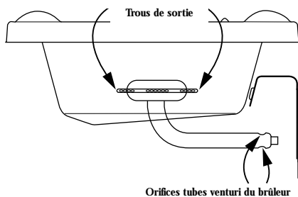
Orifices tubes venturi du brûleur
