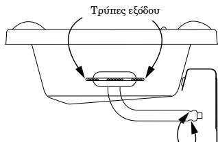
Στόμια σωλήνα venturi του καυστήρα
